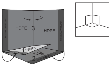
2. Ułożenie łaty w narożniku wklęsłym
