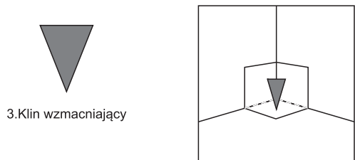
4. Wklejenie klina w narożnik wklęsły
